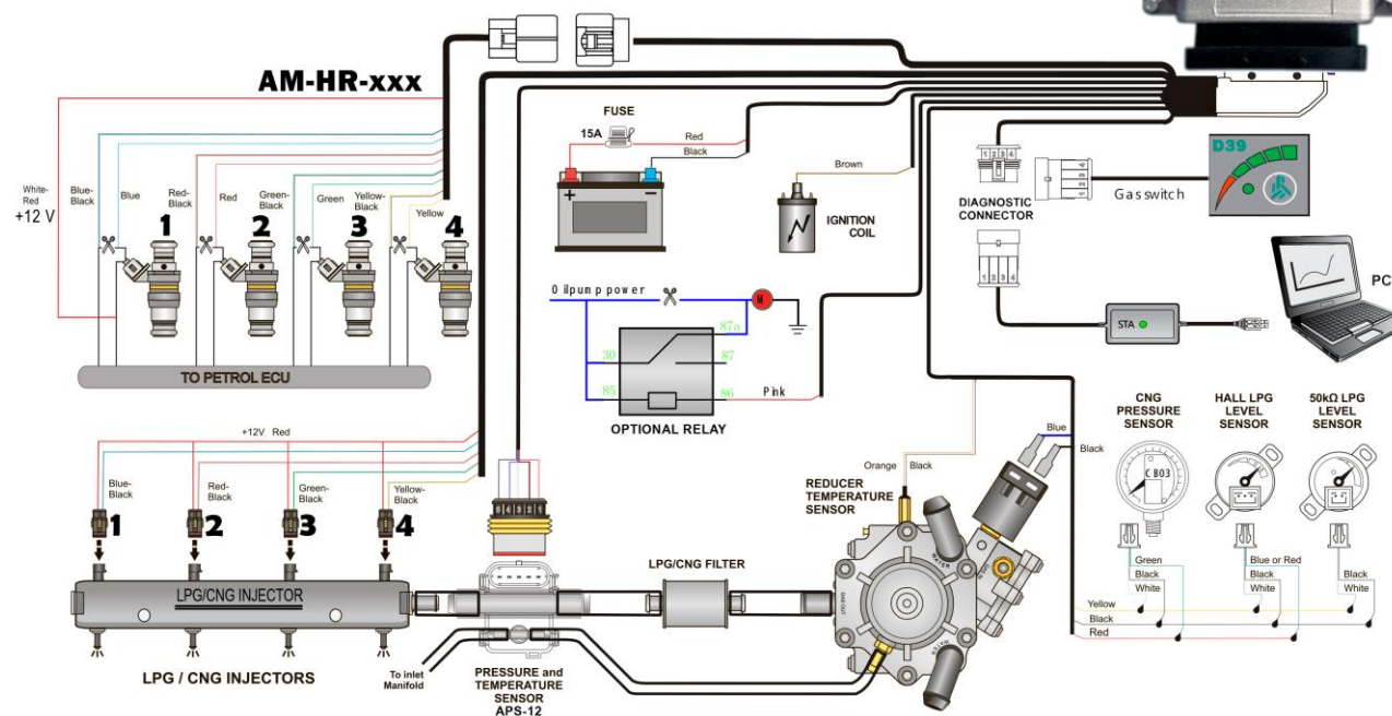
МОНТАЖНАЯ СХЕМА ALPHA D39
